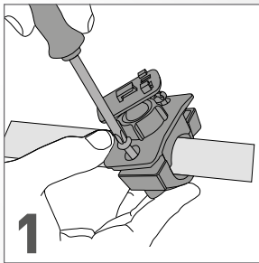
1 Sistema di montaggio. Avvitare al tubolare manubrio
