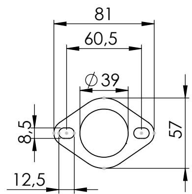
S.S. Flange 25B P/N 200560
