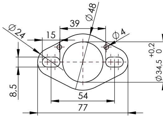
S.s. Flange Cod.206443R
