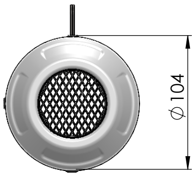
S.s. end cup set cod.309746701R
